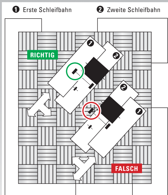
Darstellung des Schleifbahnversatzes
